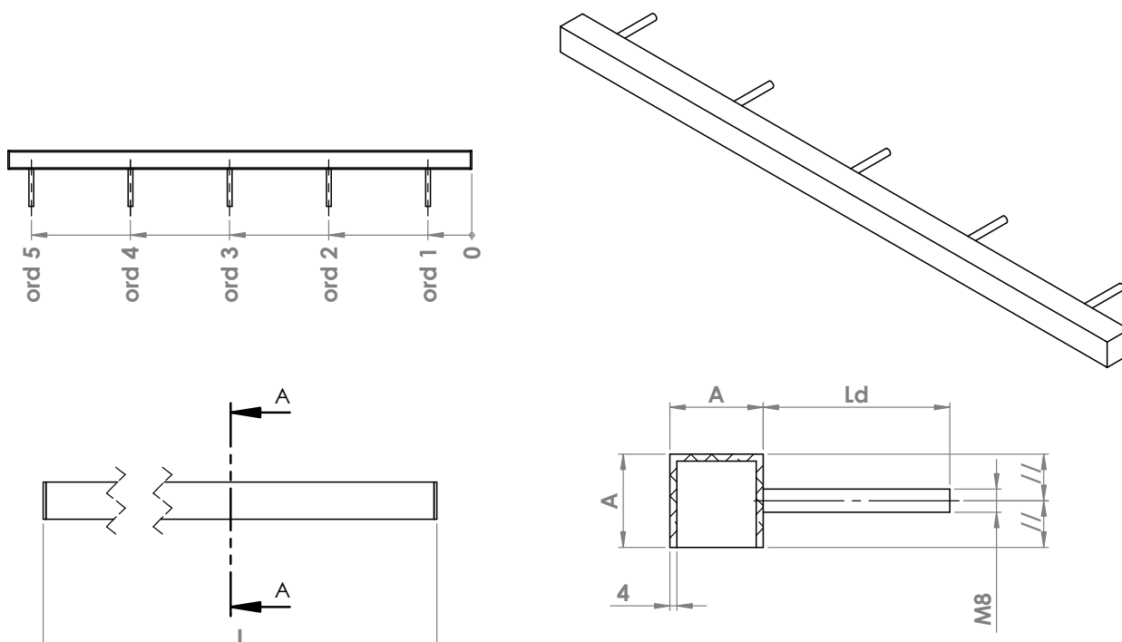
SECTION A-A SCALE 1 : 2
